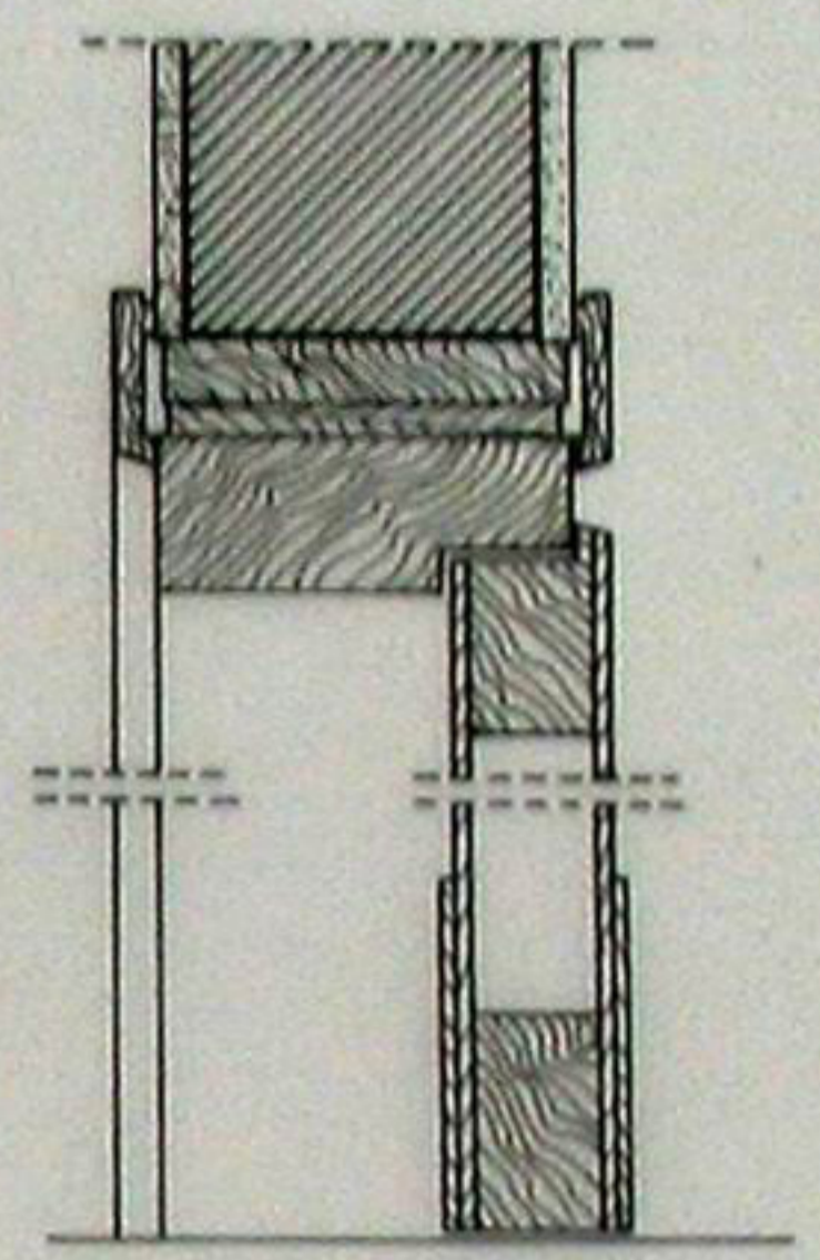
SEZIONE VERTICALE 1:4
