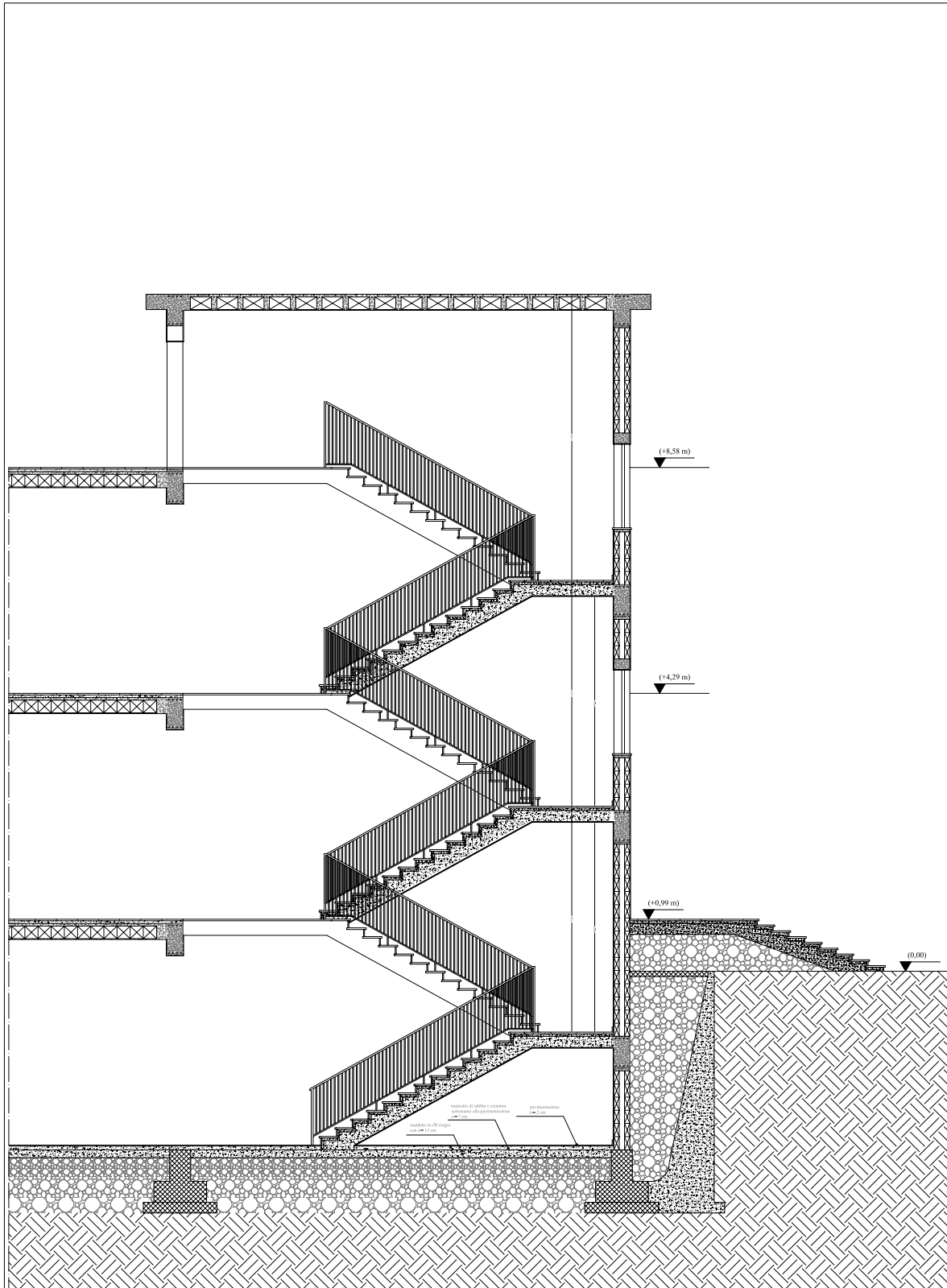
PARTICOLARE SEZIONE DELLA SCALA NEL CORPO DI FABBRICA "B" rapp. 1:20
