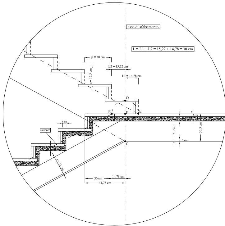
CALCOLO SFALSAMENTO DELLA SCALA CON RAMPE AL FINITO rapp. 1:5
