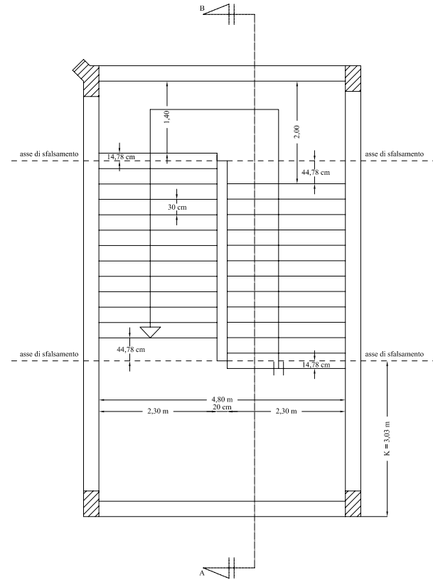
PARTICOLARE PIANTA DELLA SCALA NEL CORPO DI FABBRICA "B" rapp. 1:20
