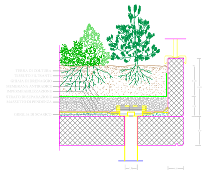
PARTICOLARE COSTRUTTIVO GIARDINO PENSILE IN SCALA ADEGUATA
